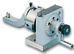
沖子成型器
