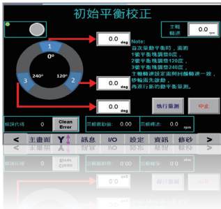
手動動平衡設定畫面 (選配功能)
