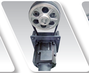
專利型伺服馬達驅動機構
