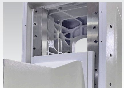
高剛性結構立柱
